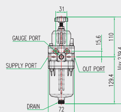
YT-220/YT-225(手动排水)
