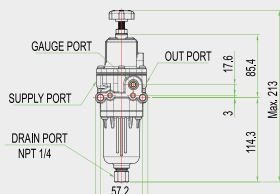
YT-200/YT-205(自动排水)
