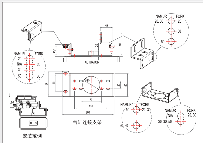
YT-1200R 系列支架
