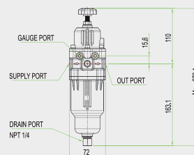
YT-220/YT-225(自动排水)
