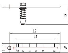
YT-3300 & YT-3350 直行程反馈杆
