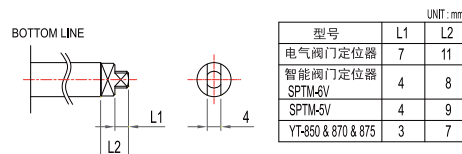
定位器角行程Namur 反馈杆
