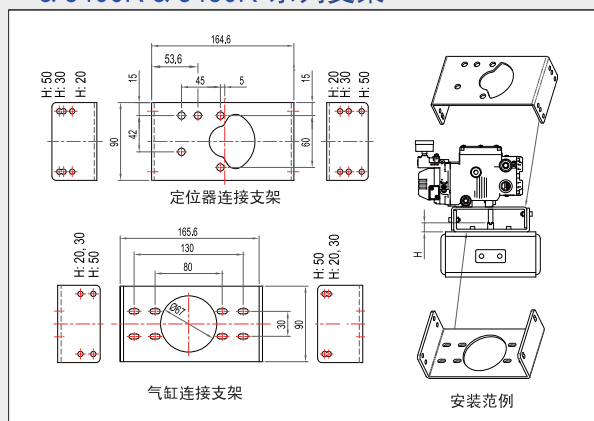
YT-2500R & 2550R & 2600R & 3303R & 3400R & 3450R 系列支架
