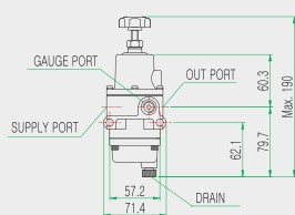
YT-200/YT-205(手动排水)
