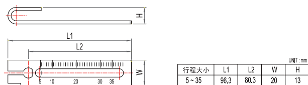
YT-2700 直行程反馈杆
