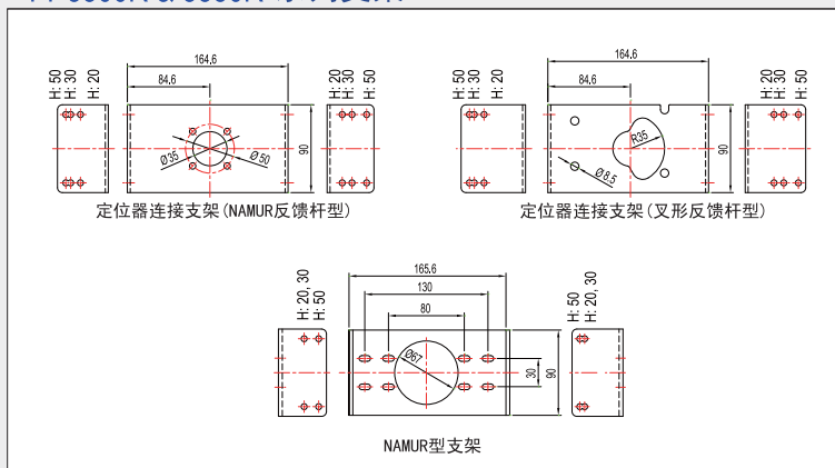
YT-3300R & 3350R 系列支架
