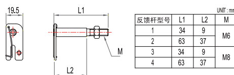
定位器角行程反馈杆
