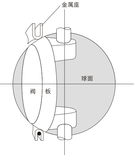
图5-1 阀板结构图
