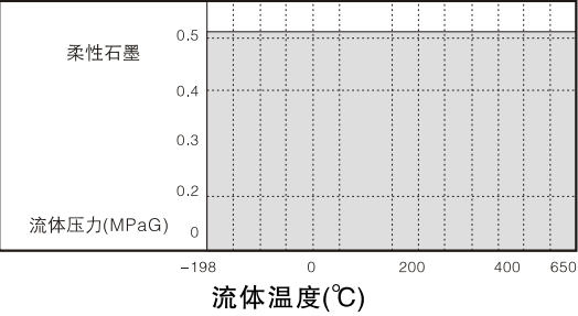
填料 使用温度、压力范围
